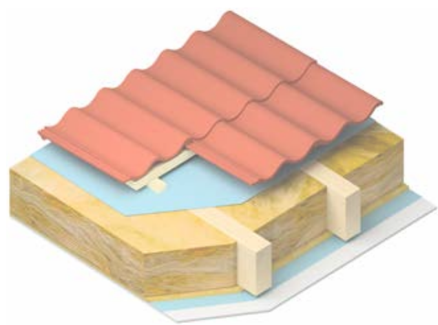
Schema der Dachkonstruktion
